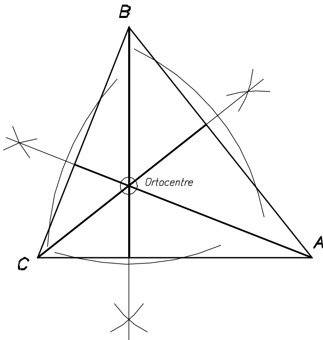
1-TRAÇAT DE LES ALTURES I OBTENCIÓ DE L'ORTOCENTRE
