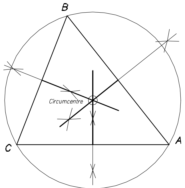
4-TRAÇAT DE LES MEDIATRIUS I OBTENCIÓ DEL CIRCUMCENTRE
