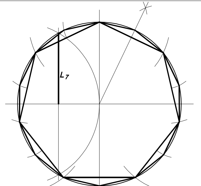
4-HEPTÀGON I POLÍGON DE 14 COSTATS (TRAÇAT APROXIMAT)
