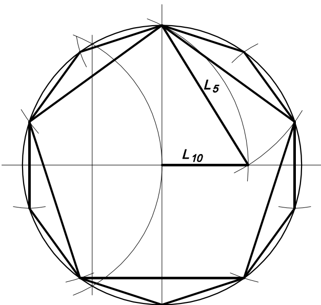
3-PENTÀGON I DECÀGON
