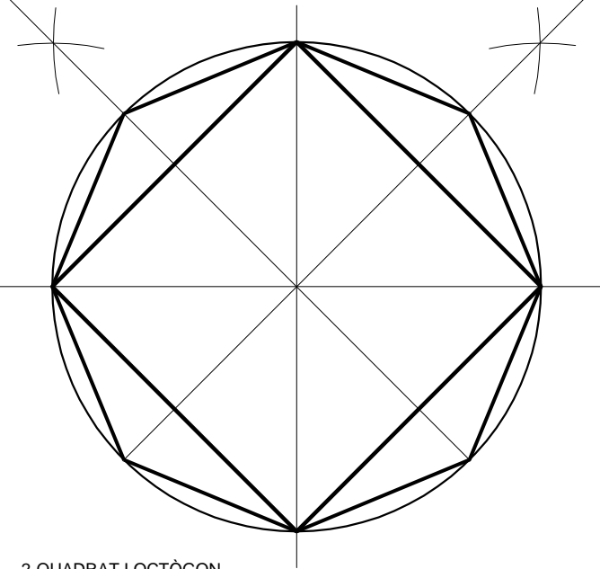
2-QUADRAT I OCTÒGON
